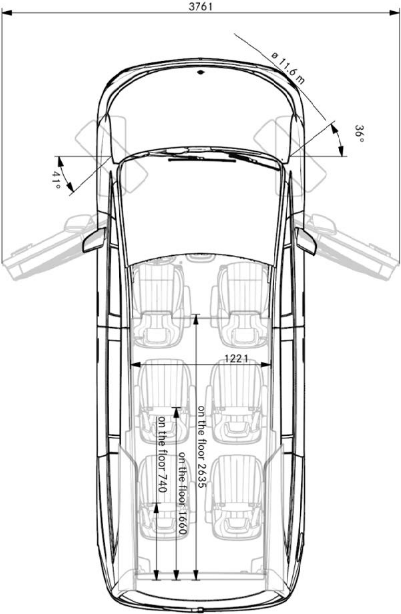
Vue dessus
