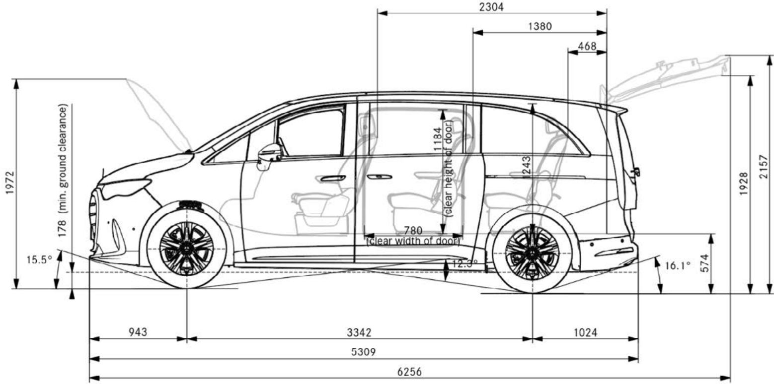
Vue latérale
